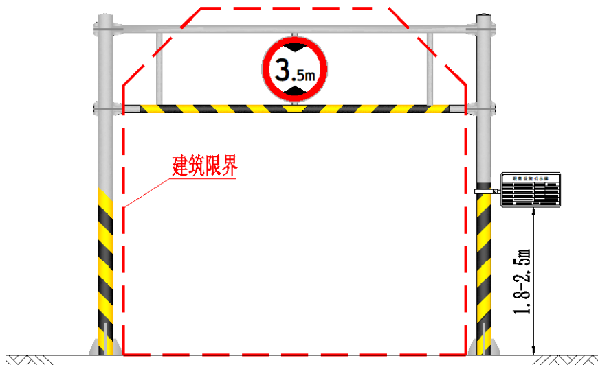
图 3 限高设施公示牌安装示例
