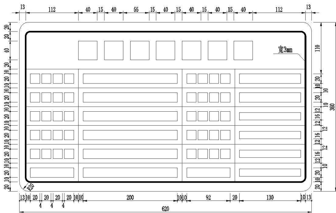
图1 限高限宽设施公示牌版面尺寸(单位:毫米)
