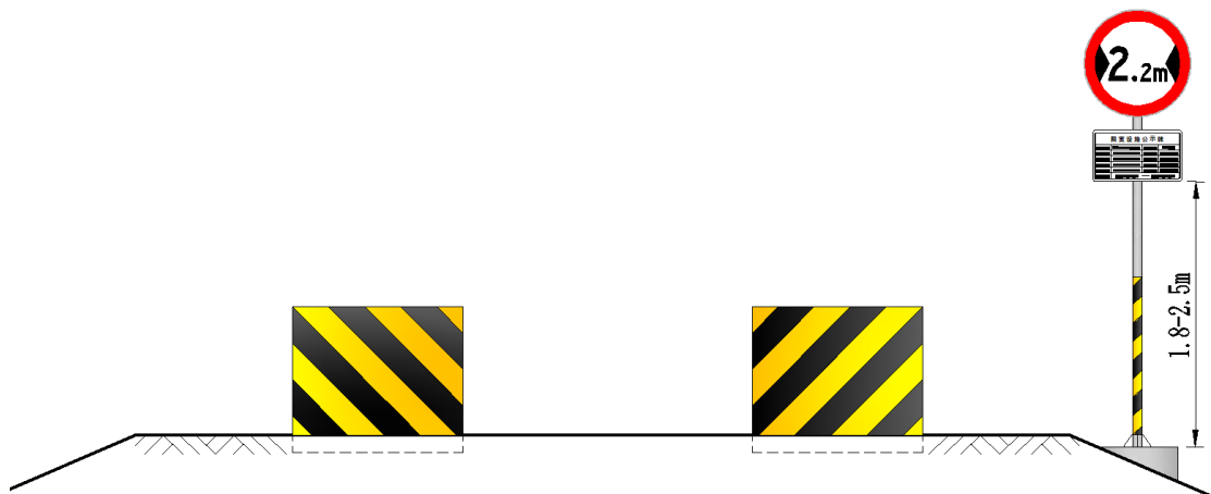
图 4 限宽设施公示牌安装示例
