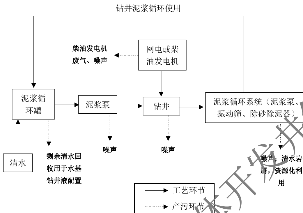
图 2.3-2 导管及清水钻井阶段及产污环节示意图
