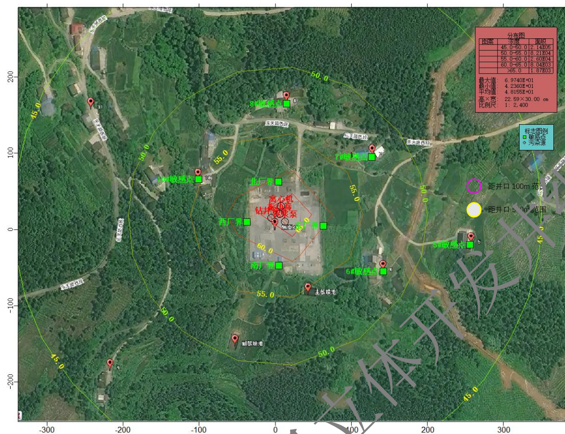
图 8.1-1 焦页 49 号平台使用网电供电时等声值线图
