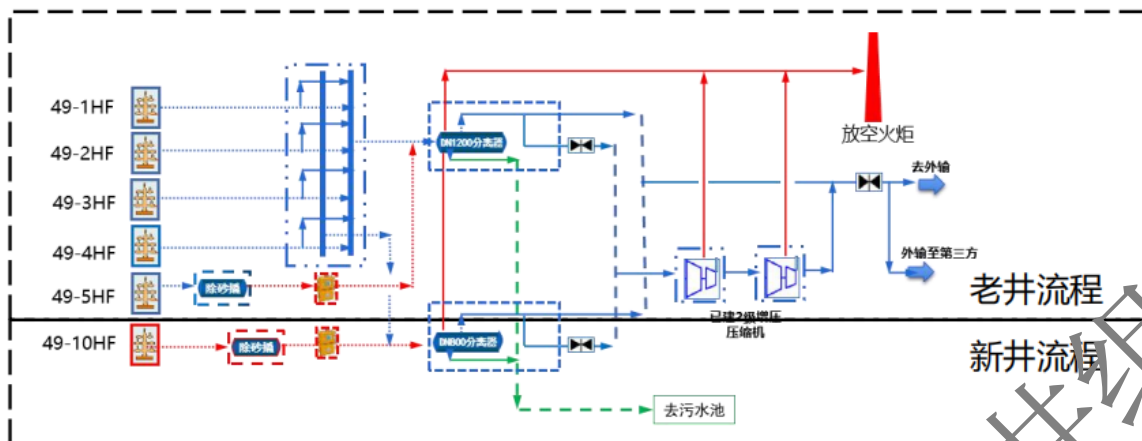
图 2.2-3 焦页 49 号集气站改造后工艺流程图
