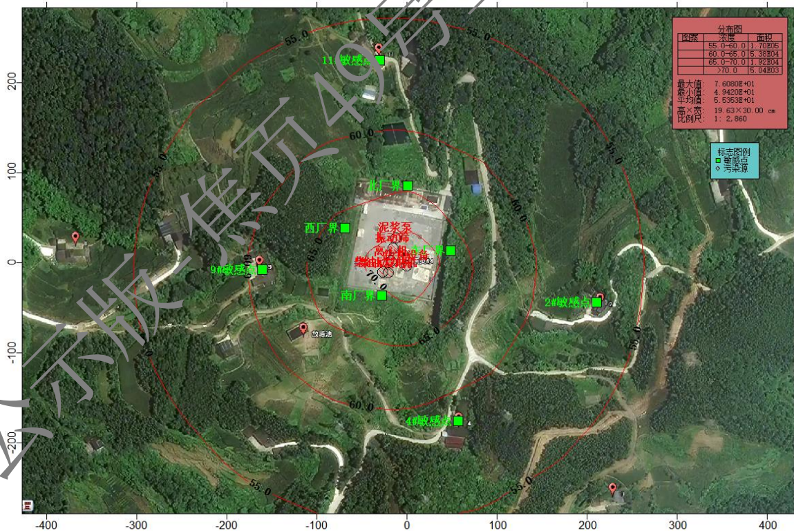
图 8.1-6 焦页 54 号平台使用柴油发电机供电时等声值线图
