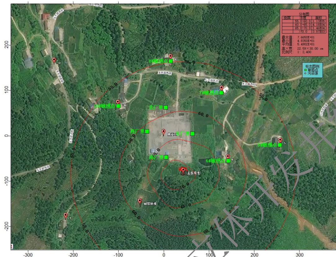
图 8.1-8 焦页 49 号平台试气等声值线图
