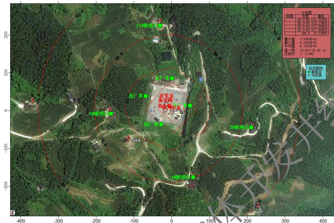
图 8.1-5 焦页 54 号平台使用网电供电时等声值线图
