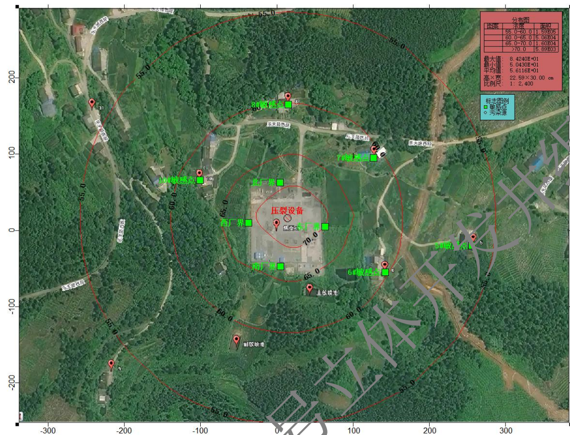
图 8.1-7 焦页 49 号平台储层改造等声值线图
