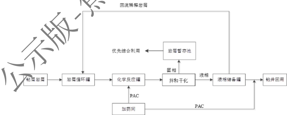
图 12.1-5 岩屑不落地系统工艺流程图
