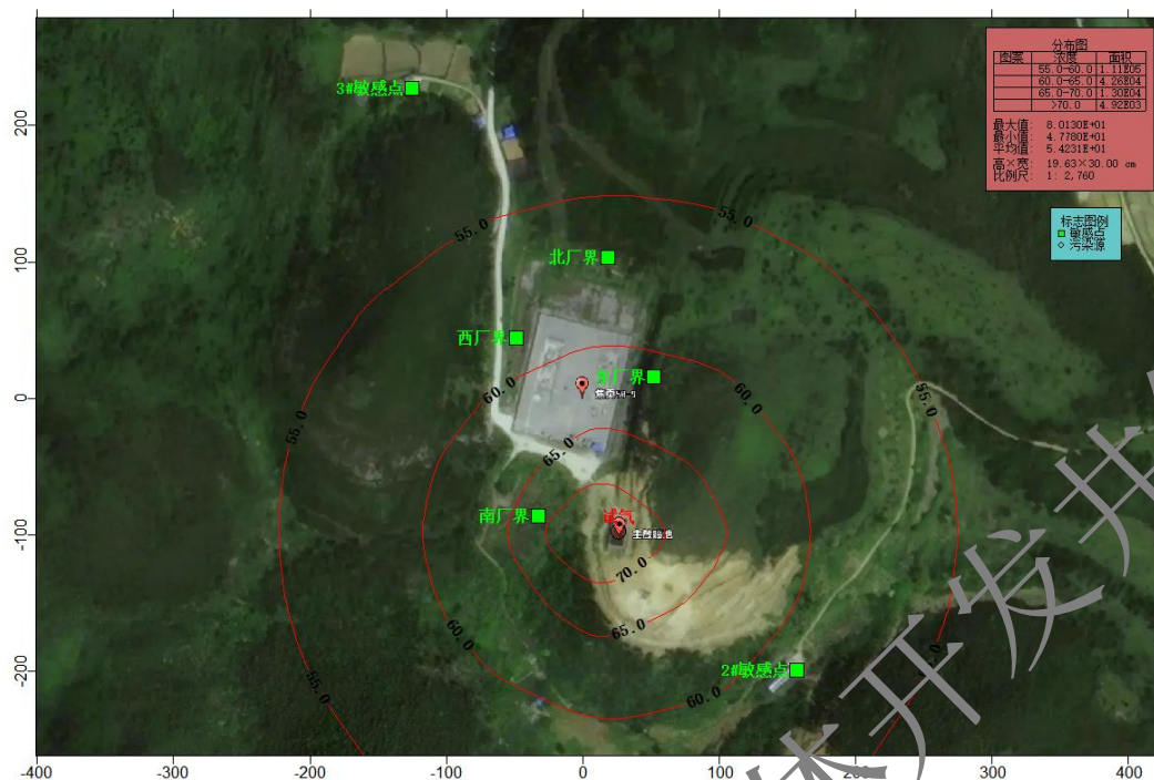
图 8.1-10 焦页 50 号平台试气等声值线图
