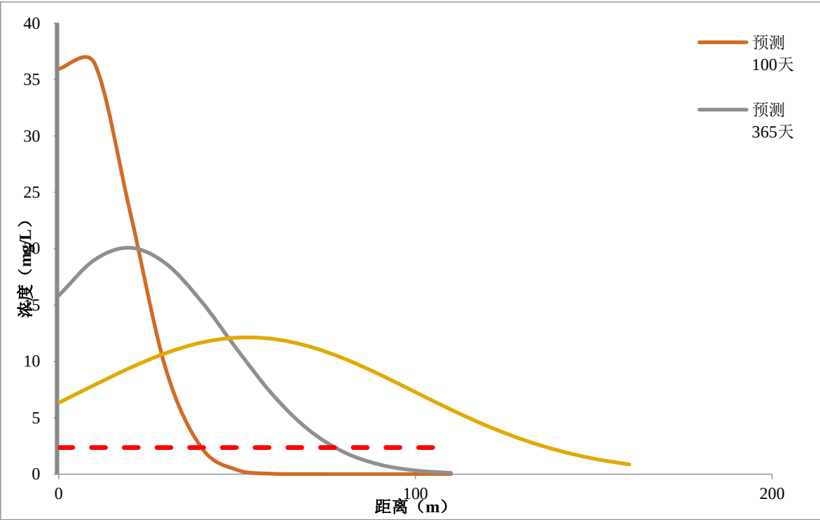
图 6.2-3 废水池漏失石油类随时间变化关系
