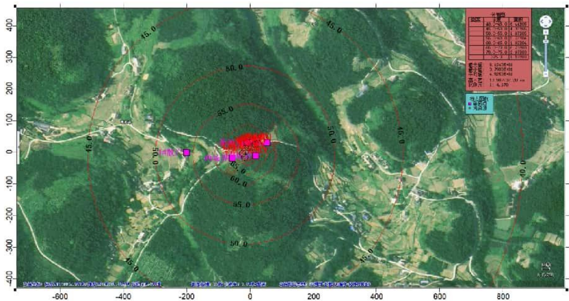
图 8.1-4 焦页 49 号北平台使用柴油发电机供电时等声值线图
