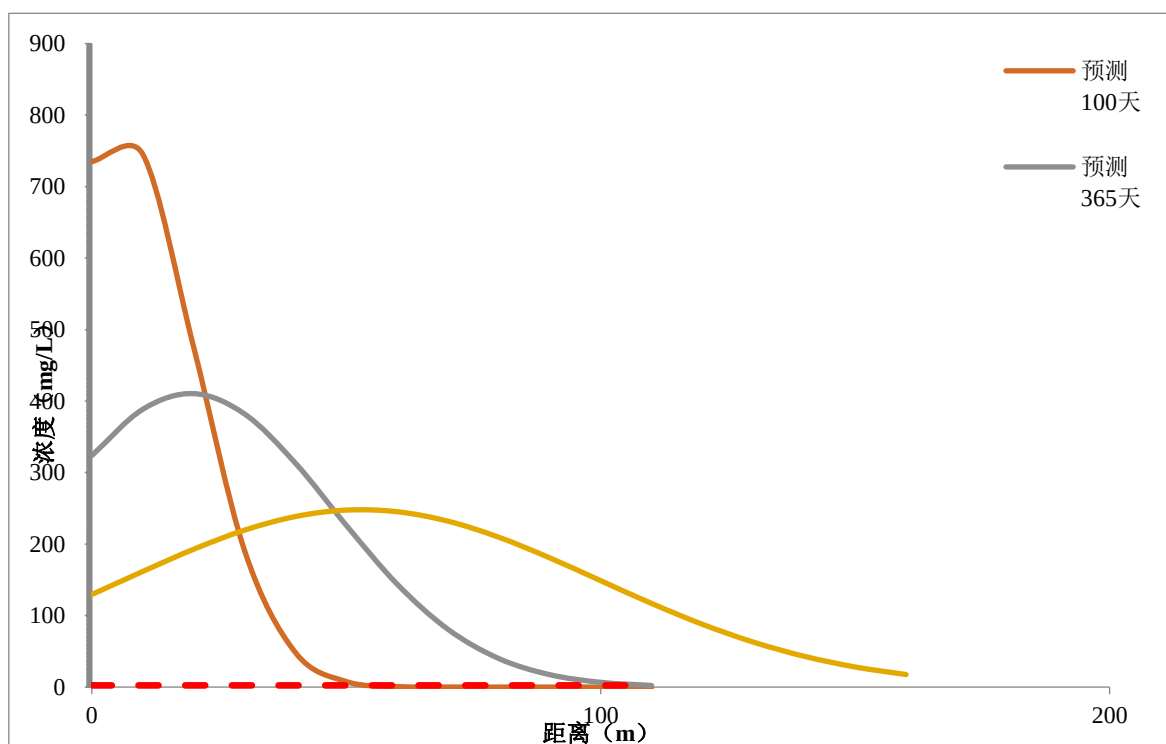
图 6.2-4 废水池漏失钡随时间变化关系
