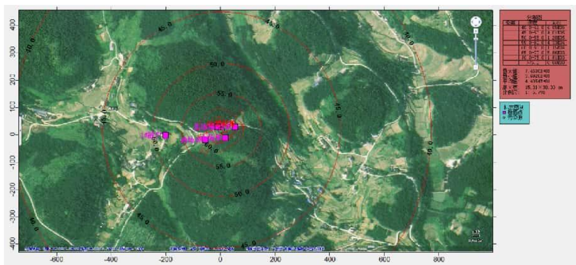
图 8.1-9 焦页 49 号北平台储层改造等声值线图
