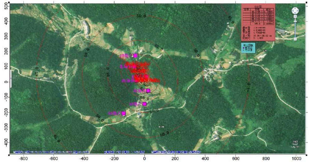
图 8.1-2 焦页 40 号北平台使用柴油发电机供电时等声值线图
