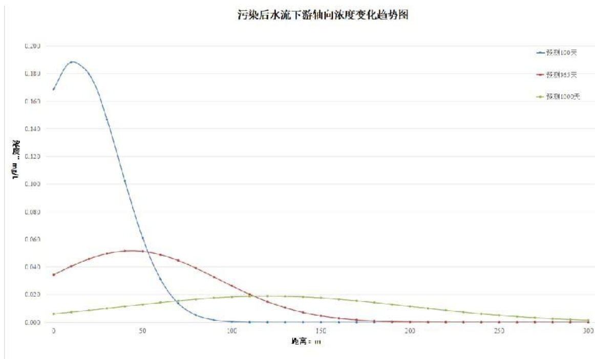
图 6.1-6 钻井液漏失石油类随时间变化关系
