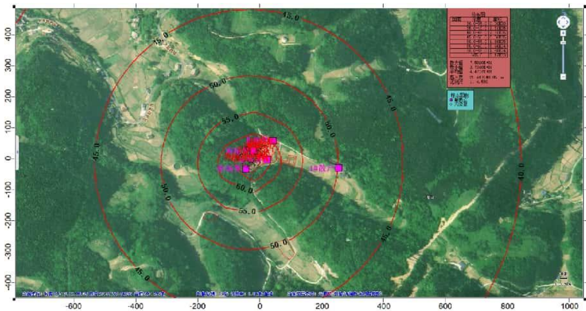
图 8.1-6 焦页 54 号北平台使用柴油发电机供电时等声值线图
