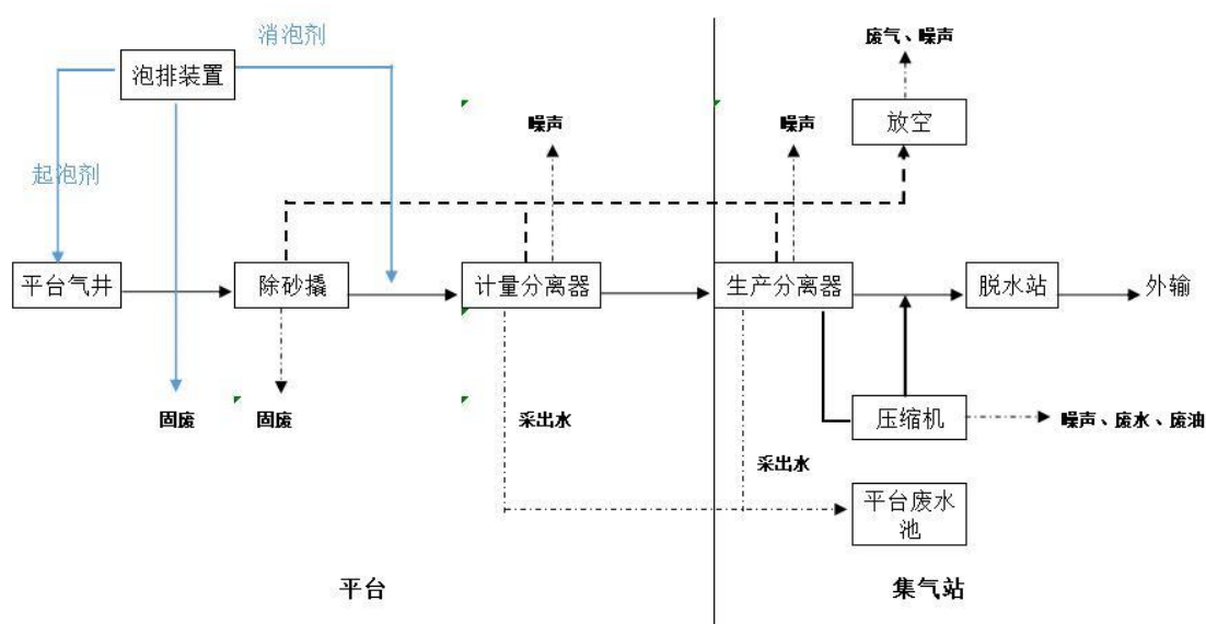
图 2.3-9 项目集输及产污节点示意图
