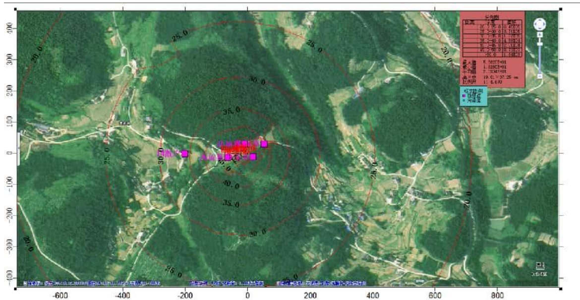
图 8.2-2 焦页 49 号北集气站敏感点噪声预测示意图
