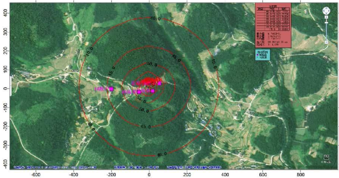
图 8.1-4 焦页 49 号北平台使用网电钻井供电时等声值线图
