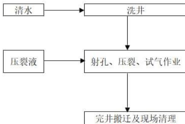
图 2.2-6 储层改造工艺流程图
