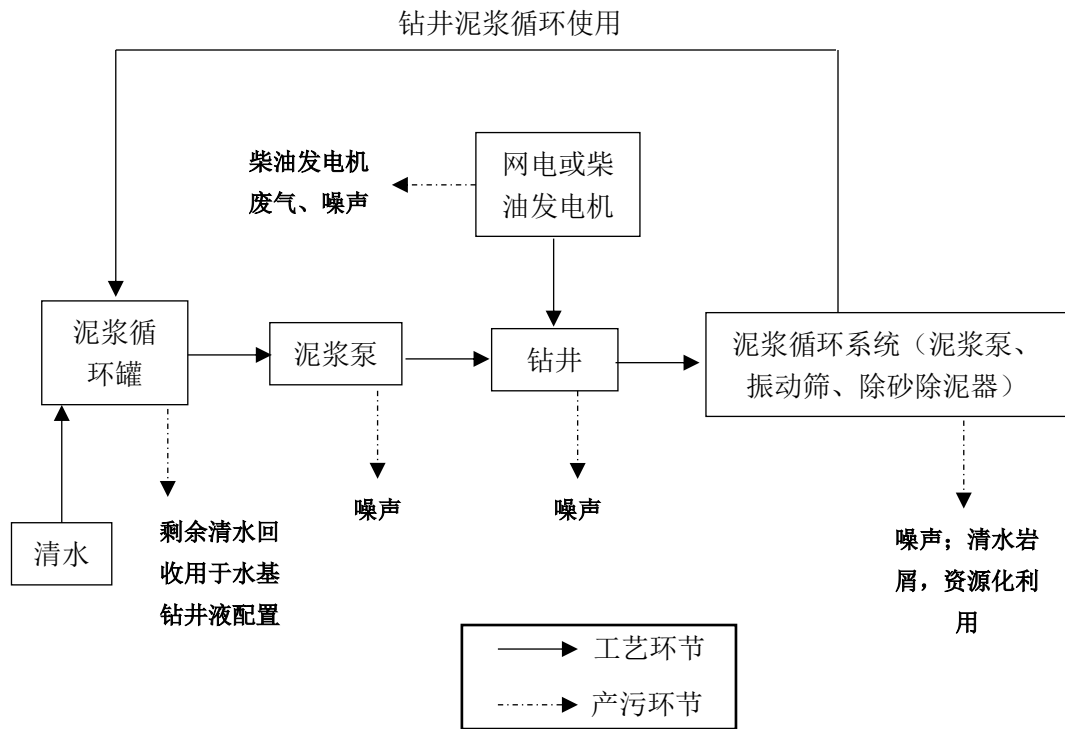
图 2.3-2 导管及清水钻井阶段及产污环节示意图
