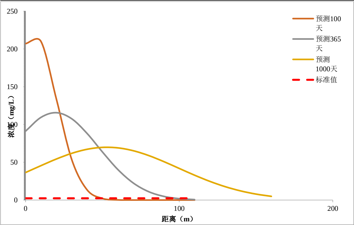
图 6.1-1 废水池漏失 COD 随时间变化关系
