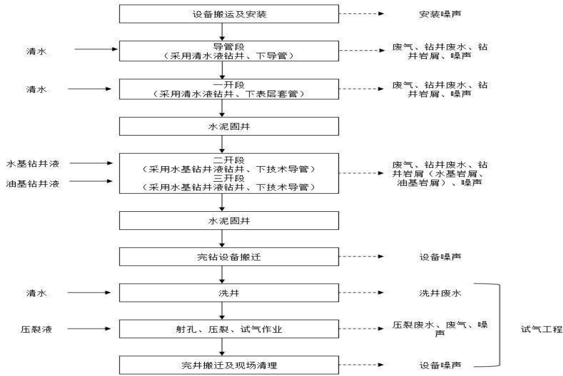
图 2.2-5 钻井作业工艺流程图
