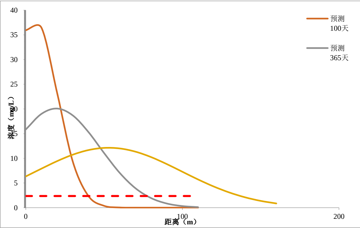
图 6.1-3 废水池漏失石油类随时间变化关系
