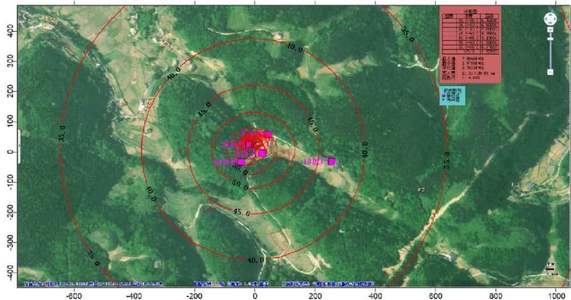
图 8.1-5 焦页 54 号北平台使用网电供电时等声值线图
