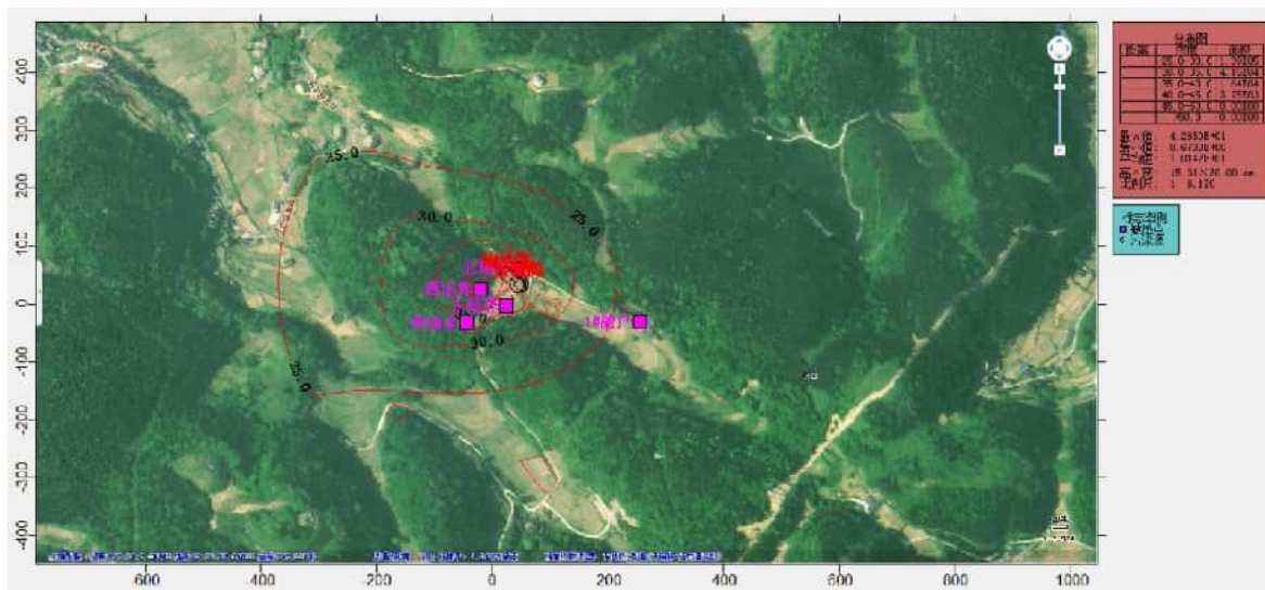
图 8.2-2 焦页 54 号北平台敏感点噪声预测示意图
