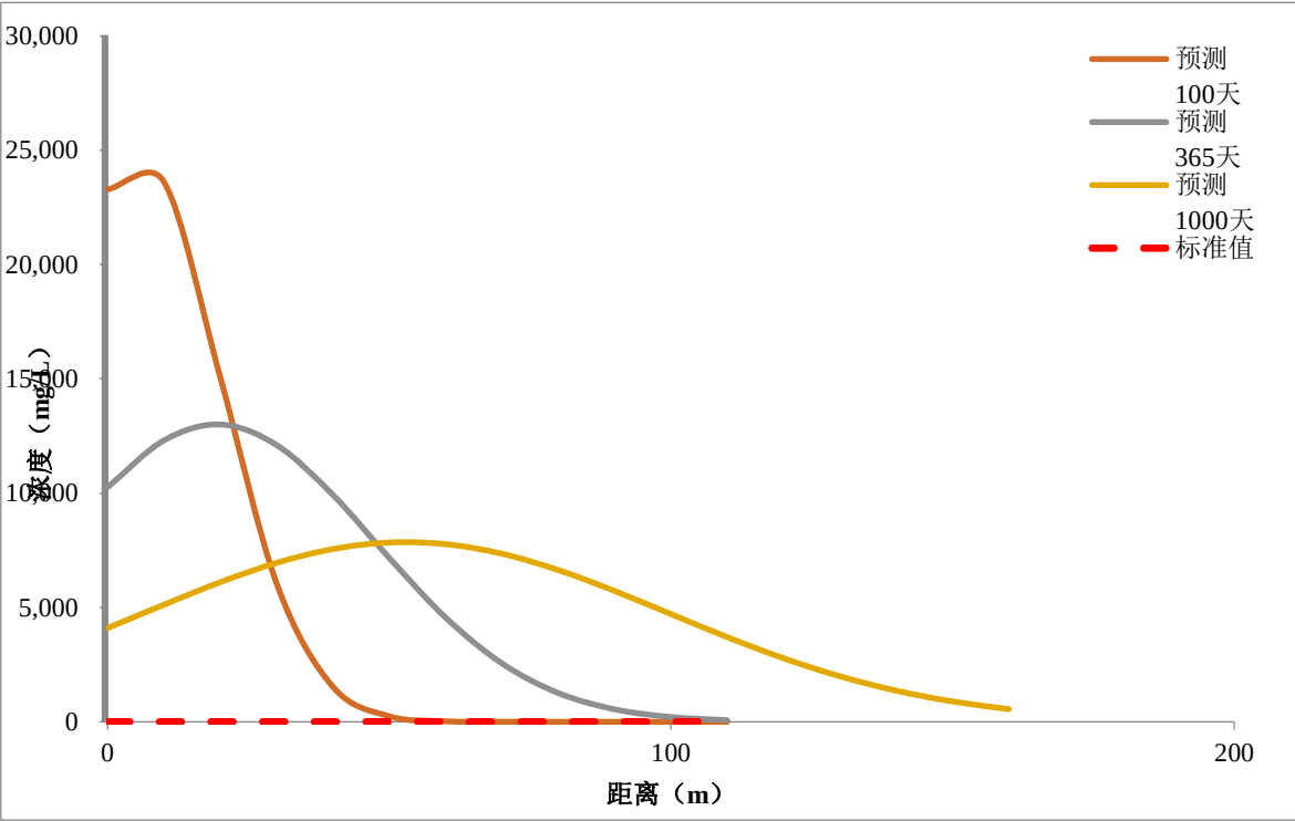
图 6.2-2 废水池漏失氯化物随时间变化关系
