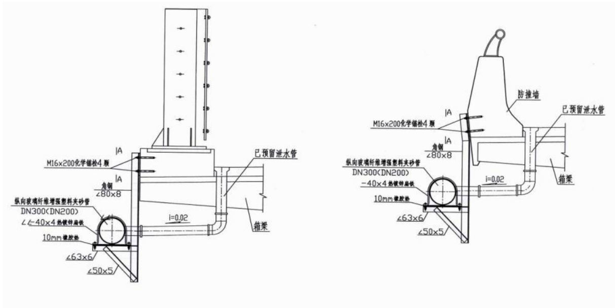
图 5.4.1-2 排水管安装示意图
