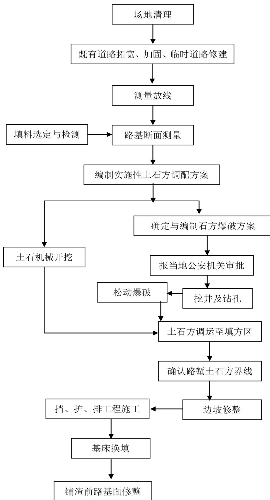
图 2.9.1-2 路堑施工工艺流程图
