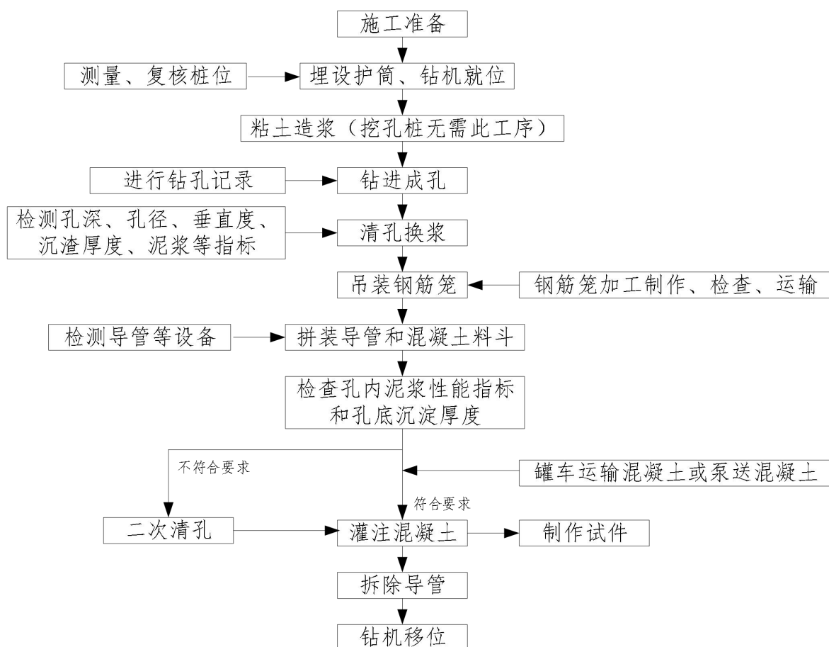
图 2.9.1-6 灌注桩施工工艺
