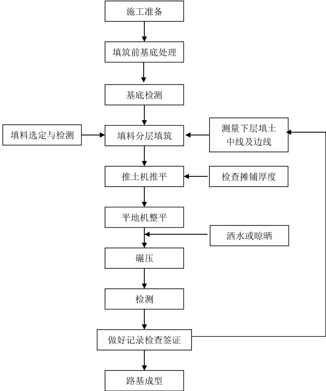
图 2.9.1-1 填筑路基施工工艺流程图
