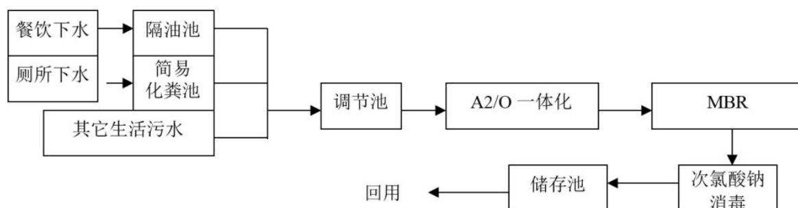
图 6.3.2-1 污水处理流程
