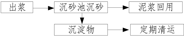
图 2.9.1-5 钻孔泥浆处置工艺
