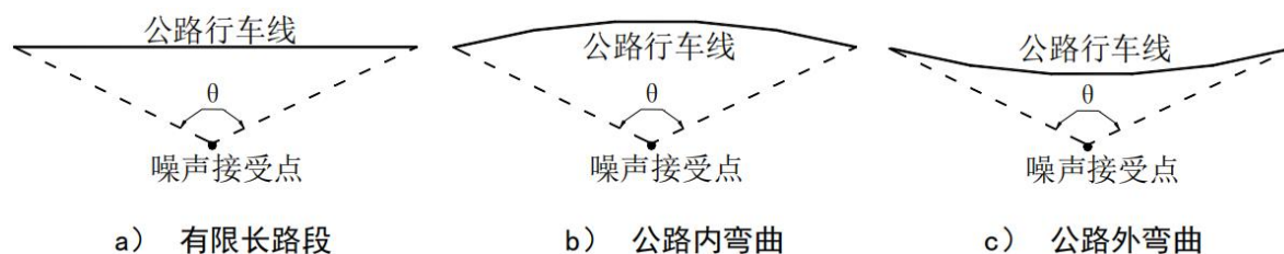
图 4.3-1 预测点到有限长路段两端的张角
