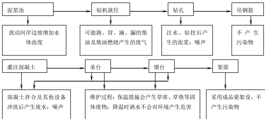
图 2.9.2-1 桥梁施工工艺流程产污环节图
