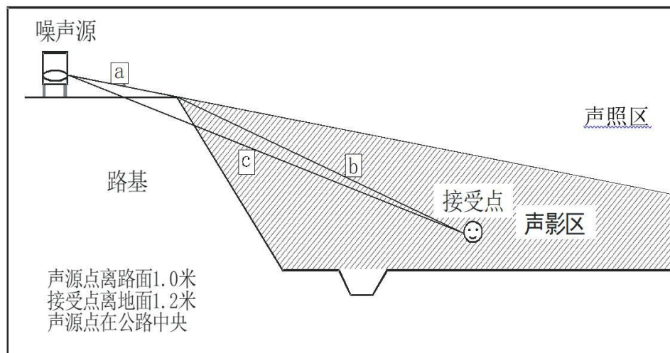
图 4.3-4 声程差 \delta 计算示意图
