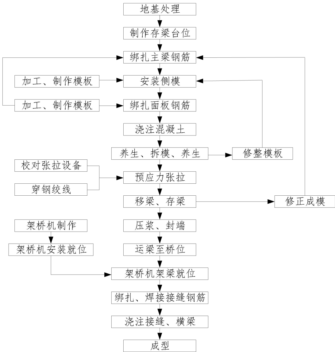
图 2.9.1-3 桥梁上部结构施工工艺
