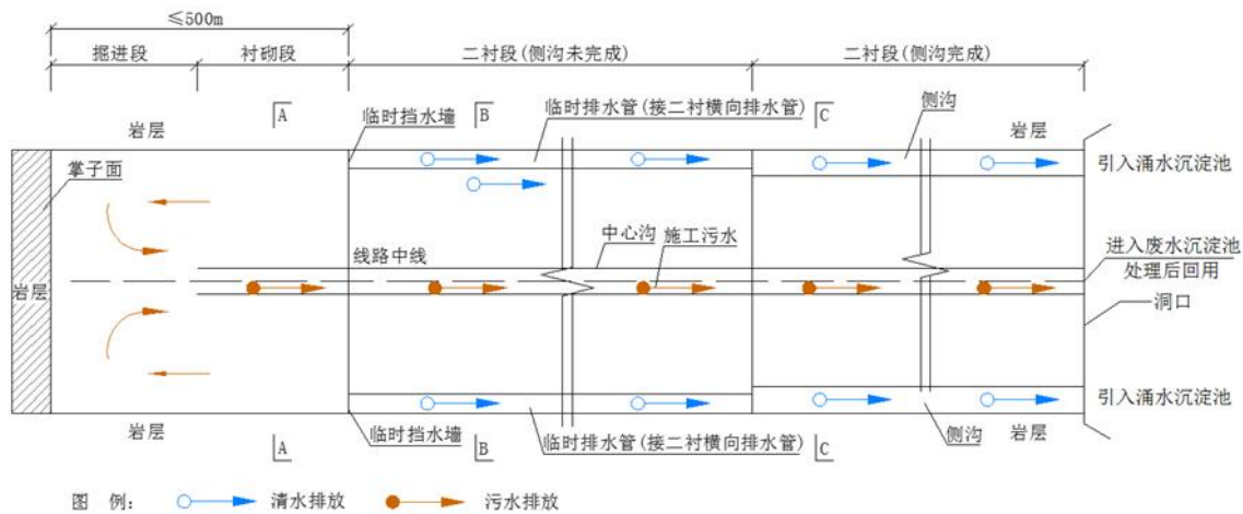
图 4.2.1-1 隧道涌水“清污分流”示意图
