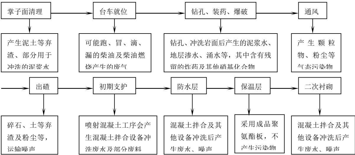
图 2.9.2-2 隧道施工工艺流程产污环节图
