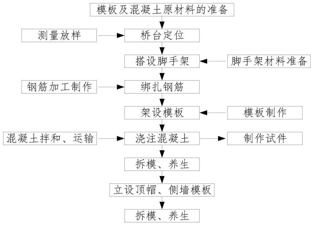
图 2.9.1-4 桥梁下部结构施工工艺
