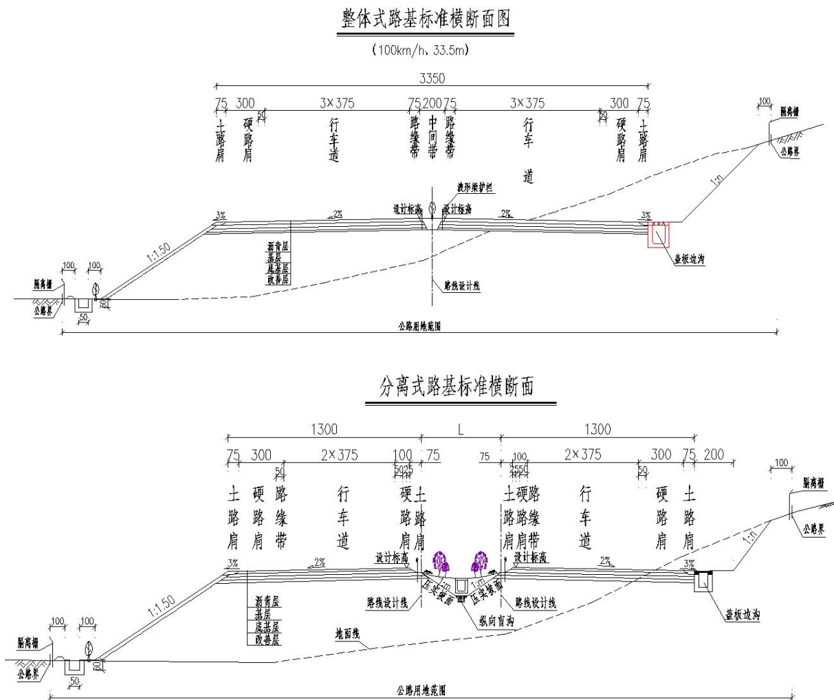
图 2.5.2-1 路基标准横断面示意图
