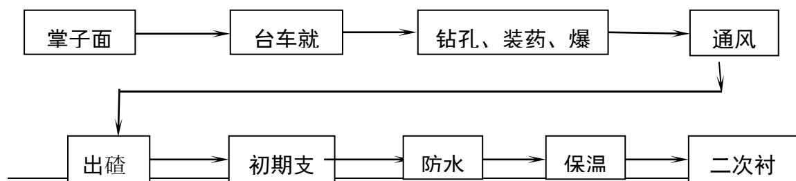
图 2.9.1-8 隧道施工工艺流程图
